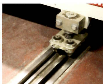
Sistema di guida a pavimento con canale incassato
