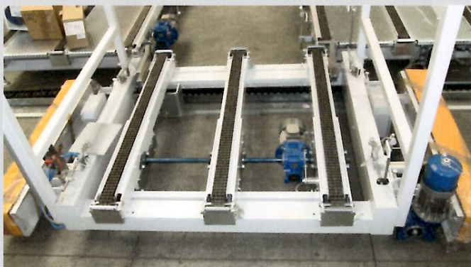
Trolley con catenaria 3 vie trasporto pallet
